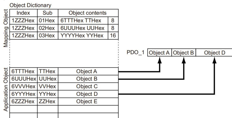
图 5-4 PDO 映射示例
