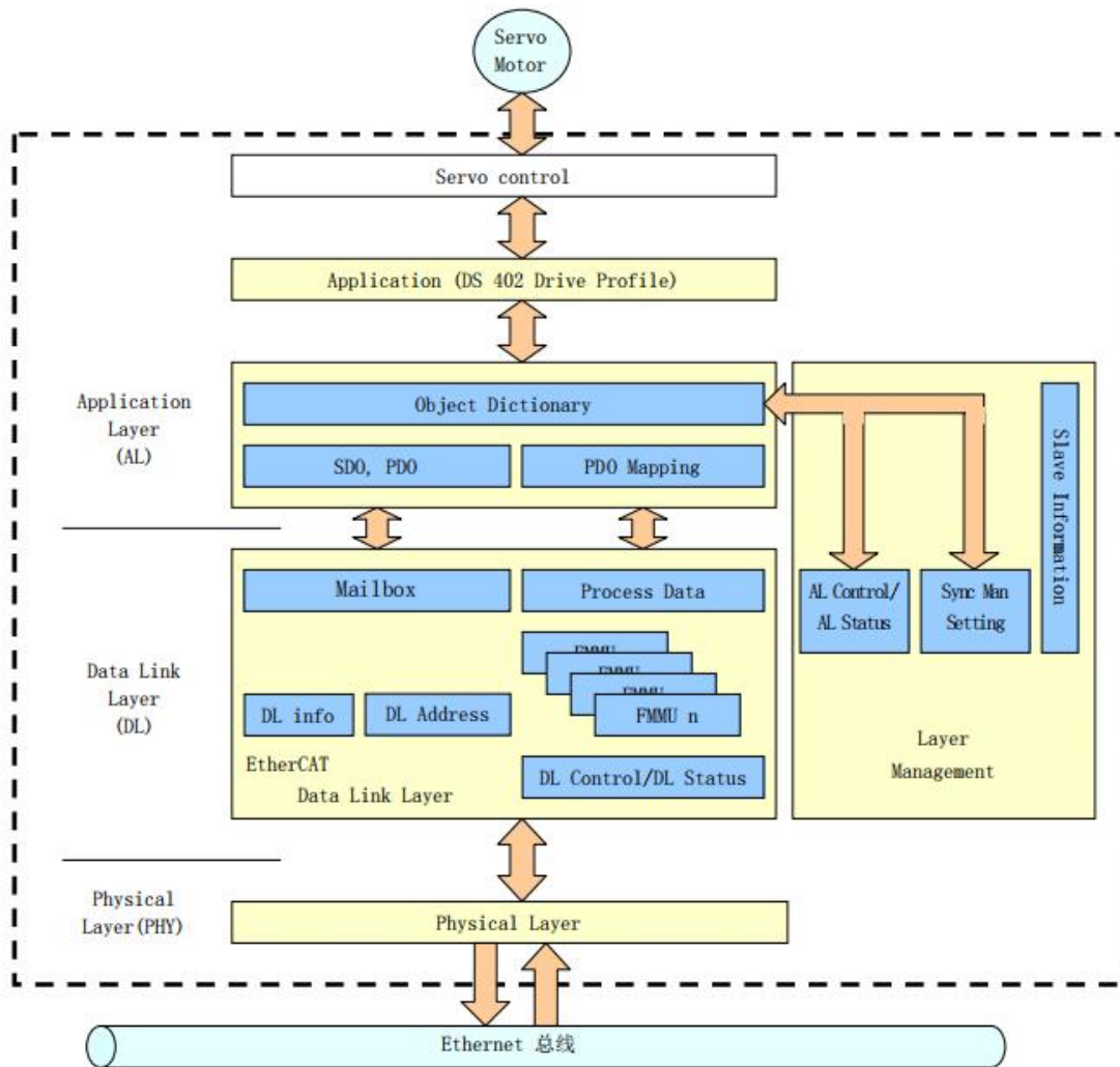
图 5-3 对象字典与设备模型
