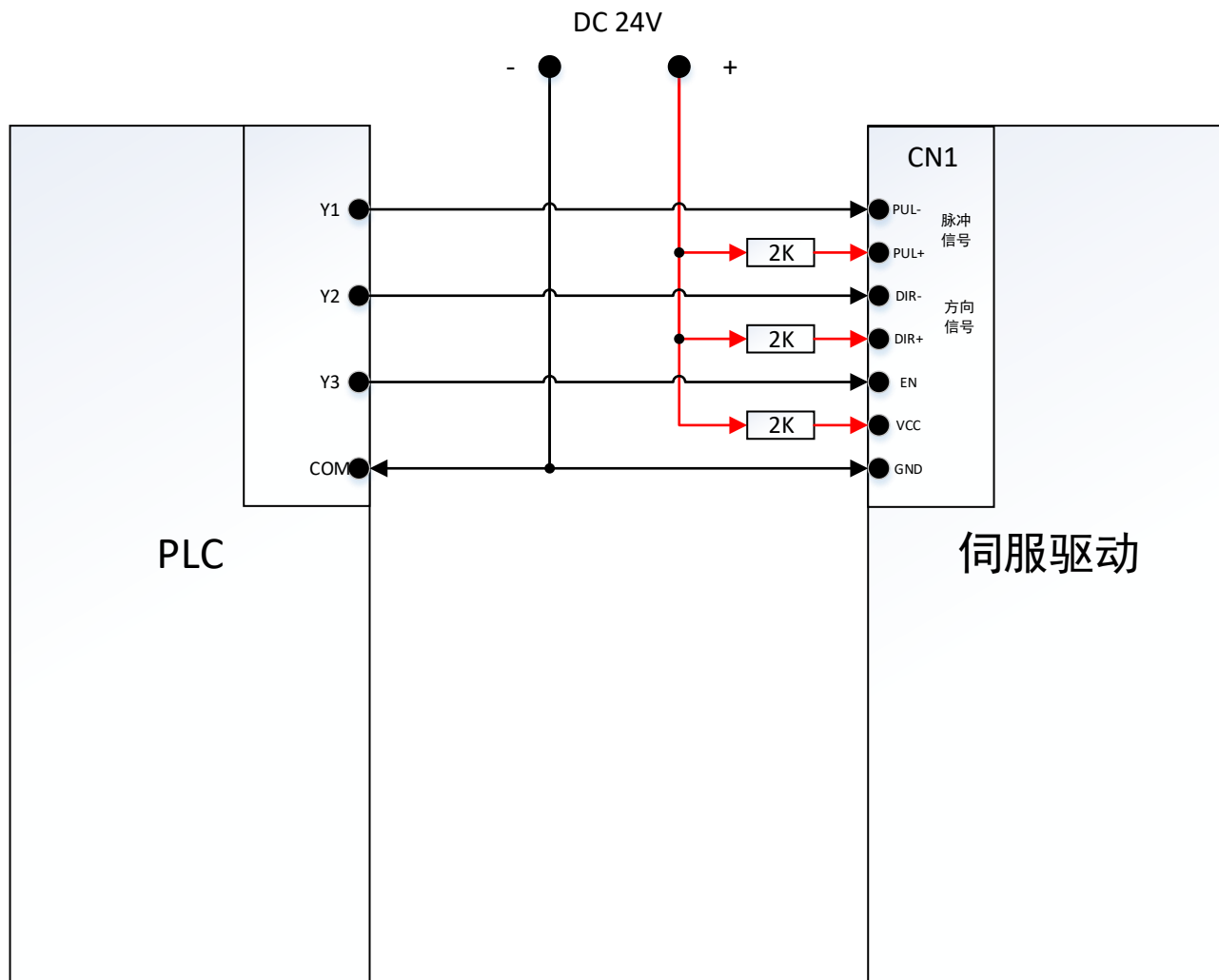
达风伺服驱动与PLC连接示意图
